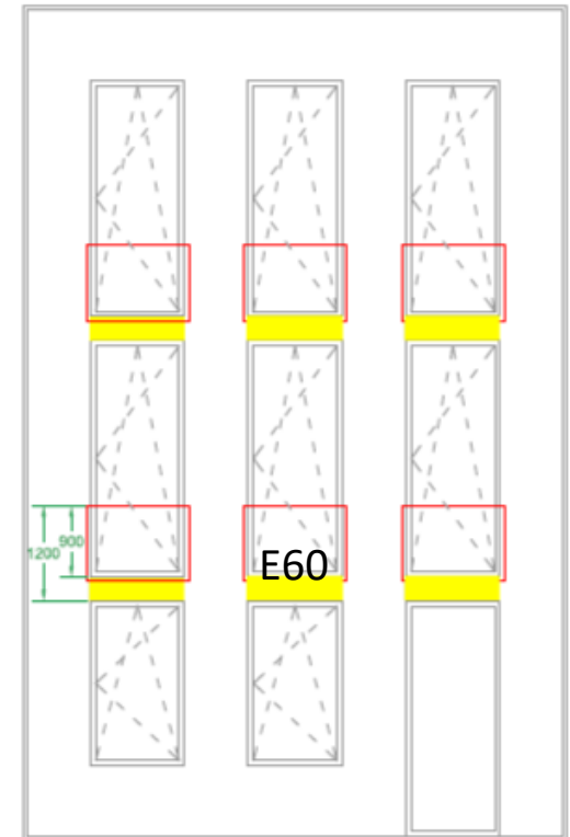
Вар.3 Остекленный междуэтажный пояс Противопожарный экран / французский балкон /
