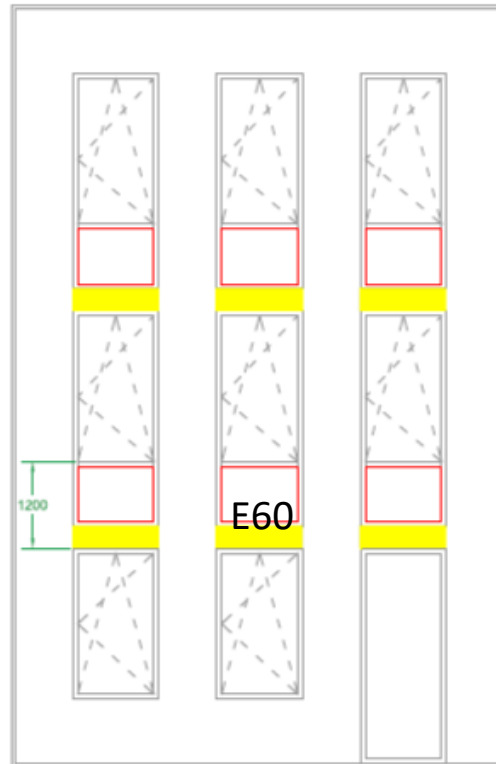
Вар.2 Остекленный междуэтажный пояс Нижняя часть окна противопожарная
